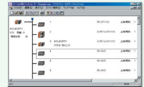
マスターパラメータ設定画面
