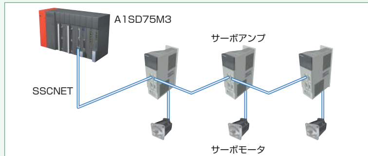
[SSCNET接続例]
