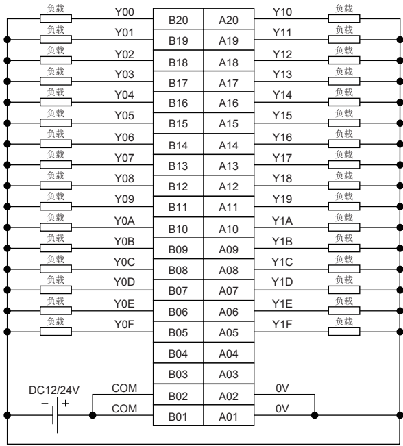
模块正面配线图
