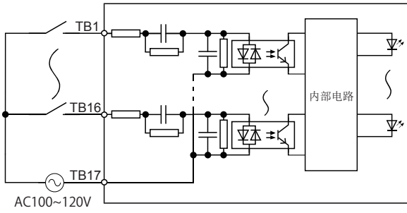
模块正面配线图
