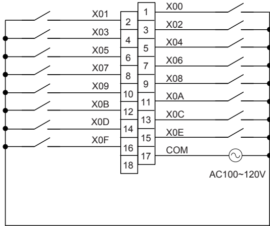
模块正面配线图
