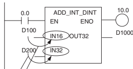
如果 IN16 为 INT 变量，则采用 D100 内容。 如果 IN32 为 DINT 变量，则采用 D200 和 D201 内容。
