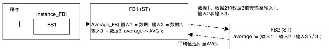
Average_FB是数据类型FUNCTION BLOCK的实例名。
